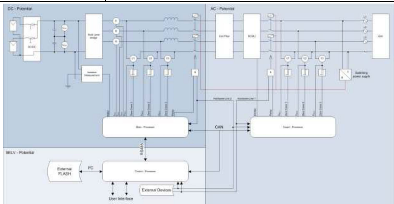
Schematischer Aufbau der Erzeugungseinheit (EZE)
