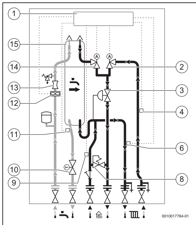
Bild 17 Funktionsschema - Station mit ungemischten Heizkreis
