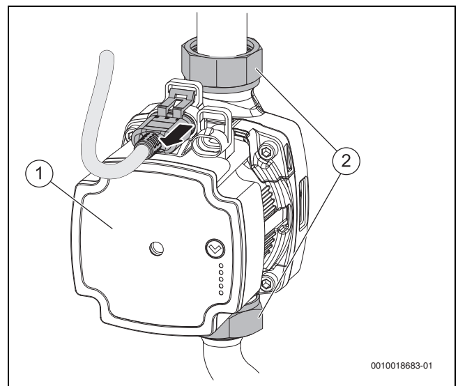
Bild 57 Heizungspumpe
