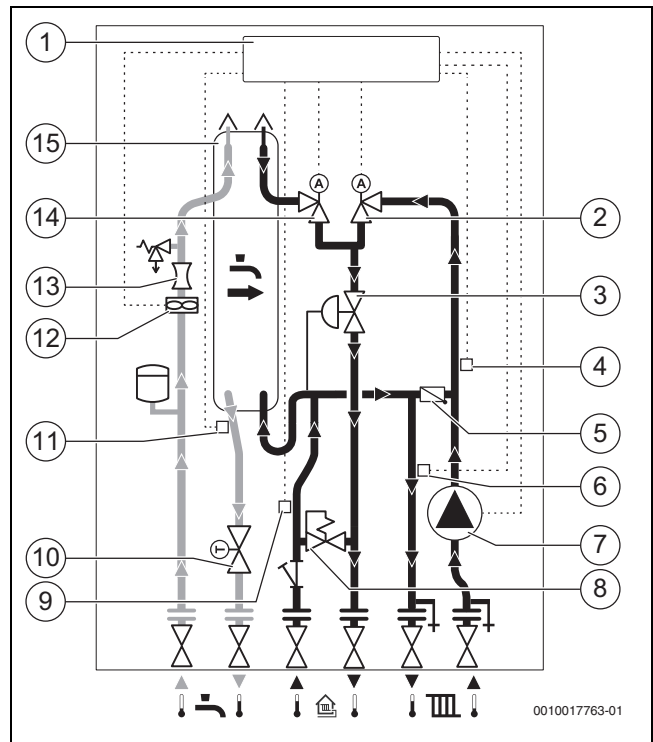
Bild 18 Funktionsschema - Station mit gemischten Heizkreis
