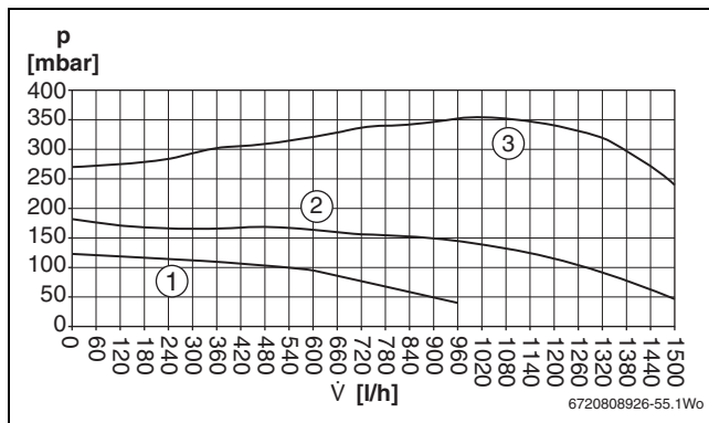
Bild 47 Restförderhöhe
