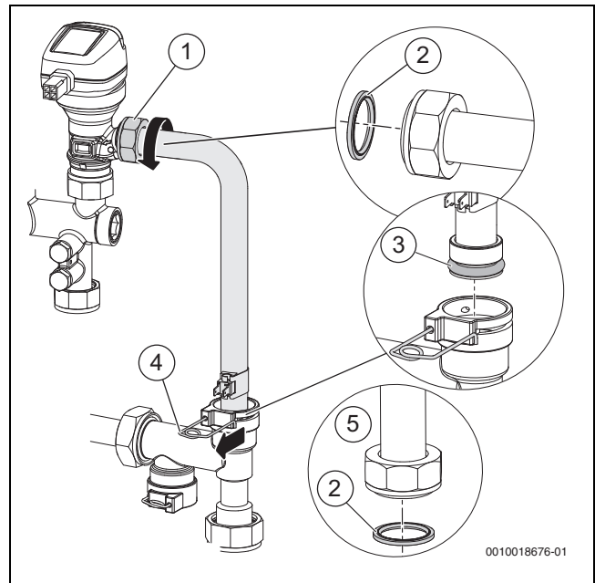
Bild 53 Rohr entfernen
