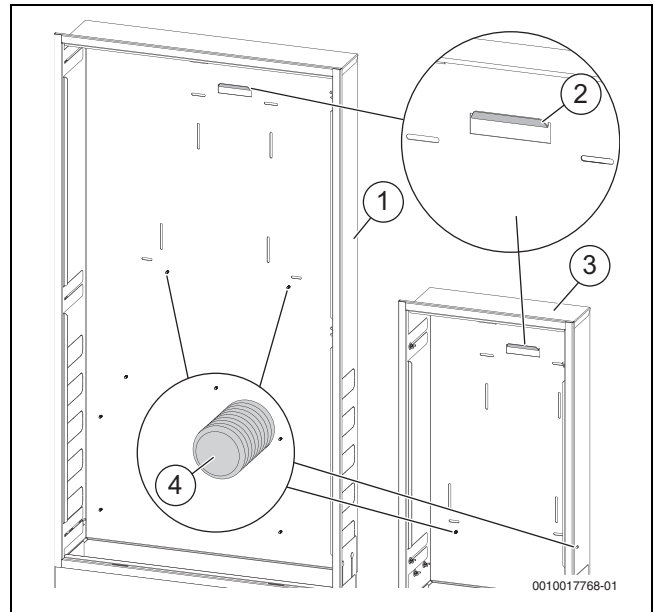
Bild 29 Unterputzkasten lang und kurz (Zubehör) Montageplatte
