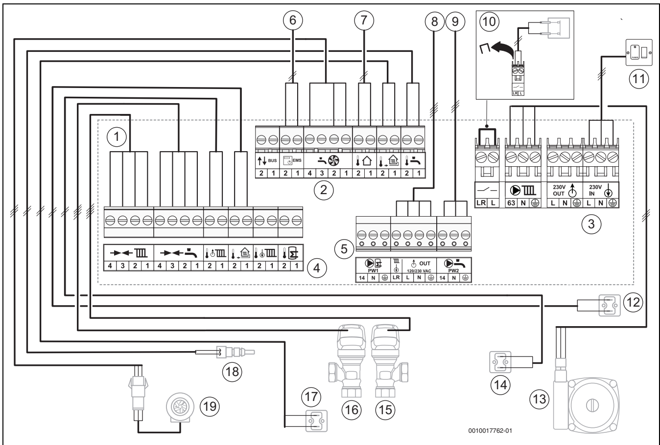
Bild 19 Schaltplan
