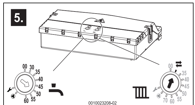
Bild 25 Drehschalter am EMS-Modul einstellen
