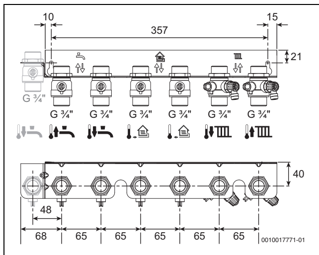
Bild 32 Montageplatte für Unterputzkasten, Maße in mm
