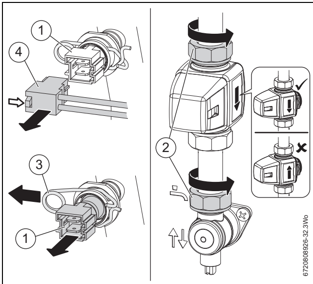
Bild 58 Warmwasser-Temperaturfühler und thermische Absicherung
