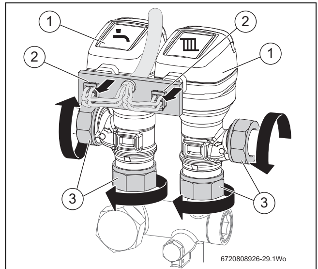
Bild 56 Regelventile
