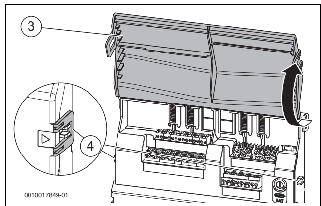
Bild 37 Abdeckung hochklappen
