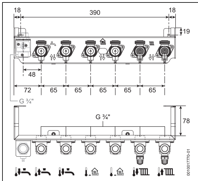
Bild 31 Montageplatte für Aufputzmontage, Maße in mm
